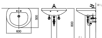
평면 붙임 세면기 DL-401
