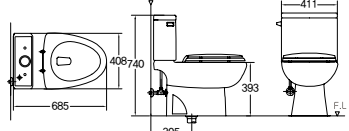
탱크 밀결형 사이펀 변기 DC-211N
