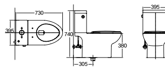
탱크 밀결형 사이편 변기
