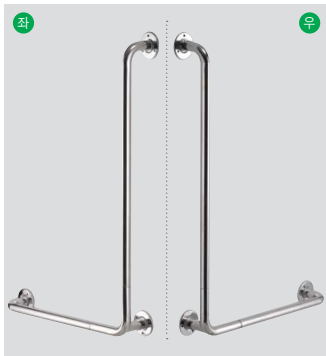
■ HL 900 L자형 (좌타입), HR 900 L자형 (우타입), HS 900 (좌우 겸용타입) · L-Type Grob Bar for a Toilet bowl · 재질: Stainless Steel · 사이즈: W600×H900 · 파이프: Ø32, Ø38
