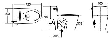
하이탱크 일체형 변기 DC-611
