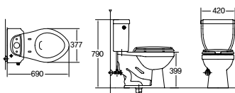
탱크 밀결형 사이펀 변기 DC-202
