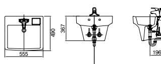
평면 붙임 일체형 세면기(비누대) DL-511SS
